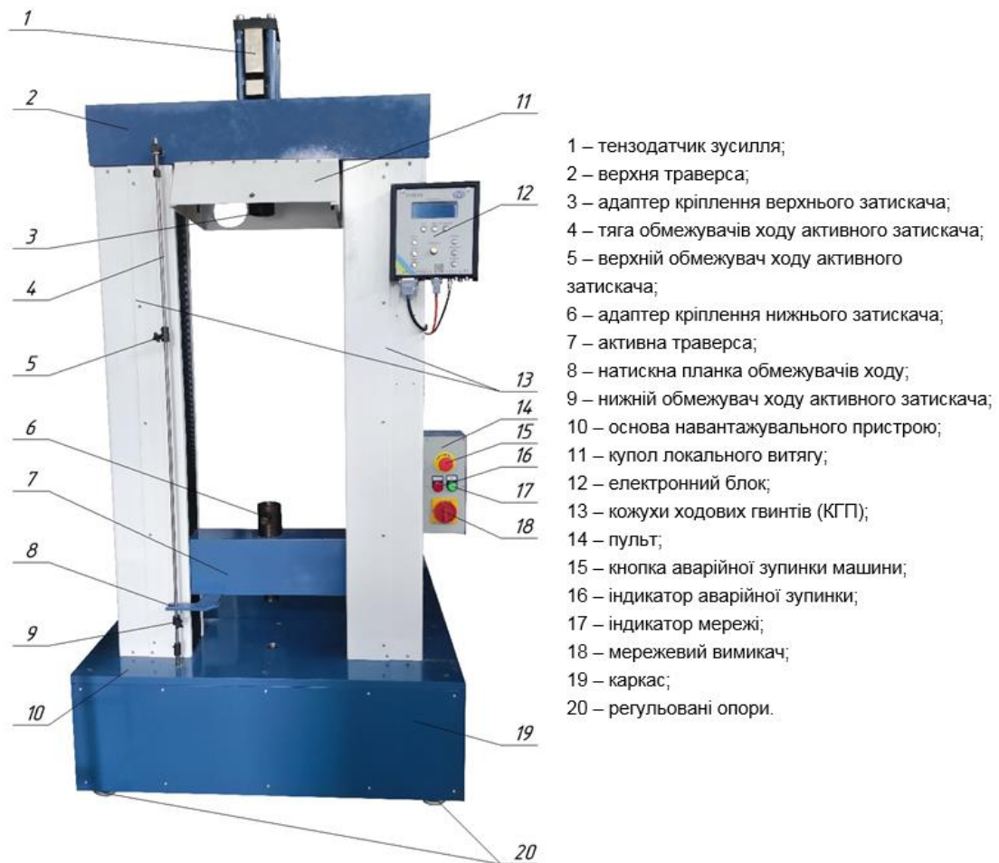
Мал. 1 – Загальний вигляд машини випробувальної МРМ-10Т
